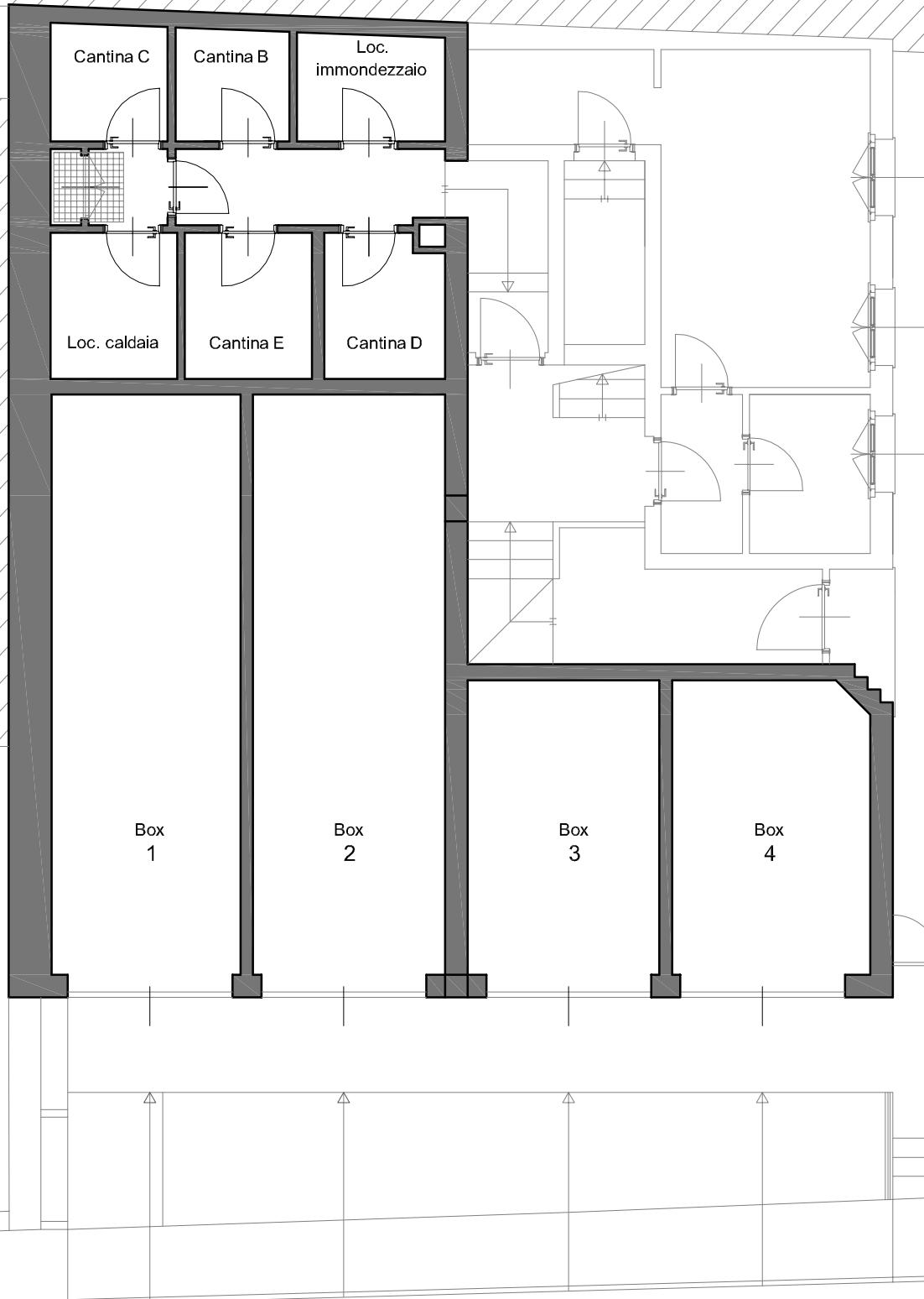
CANTINE E BOX scala 1:100
